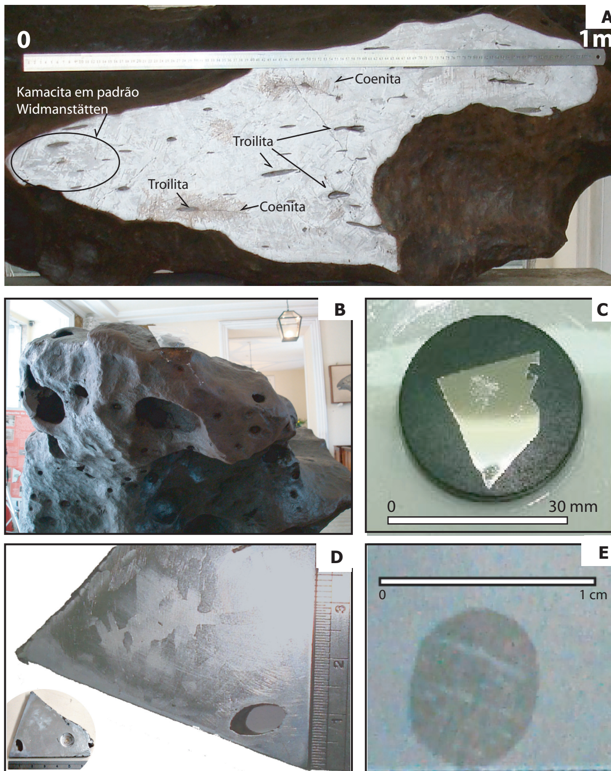
Figura IV.8. Fotos das amostras trabalhadas para a descrição petrográfica macro e microscópica do Bendegó. Massa principal exposta no Museu Nacional: (A) face polida mostrando ocorrências de troilita, coenita e kamacita com padrão Widmanstätten e (B) Face anterior (bico) com cavidades de dimensões e profundidades variadas, resultado da ablação da troilita. Amostras cedidas pelo Museu Nacional, polidas e atacadas por nital para estudos petrográficos: (C) Lâmina para microscopia eletrônica de varredura, (D) amostra triangular, (E) nódulo de troilita.
